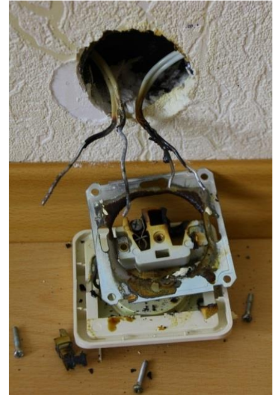
ПІДГОРІВША РОЗЕТКА
